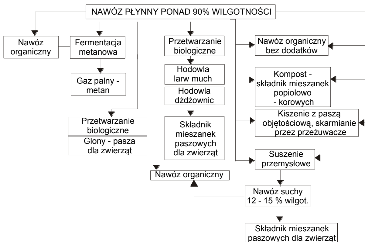
Rysunek nr 21: Sposoby wykorzystania i zagospodarowania gnojowicy w chowie bezściółkowym.
